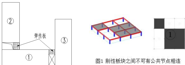
图 2.4.3 刚性板设置方式
