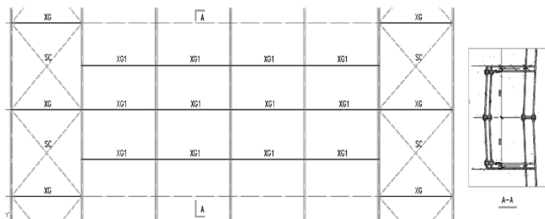
图 2.6.10 某天窗架支撑设置 (局部)
