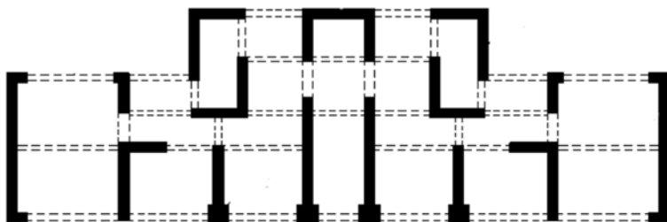
图 2.5.22 一向少墙剪力墙结构
