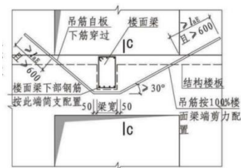
图 2.5.17-1 设置吊筋做法
