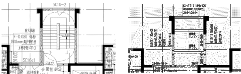
图 2.5.20 外凸楼梯间结构示例
